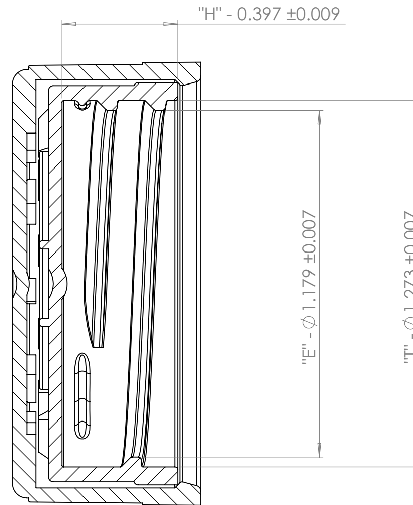
SECTION A-A
